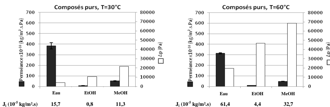
Figure 5 : Densité de flux partiel, perméance et force motrice de l'eau, éthanol et méthanol purs dans le cas de la membrane Hyb-Si® (IC à 95 %)
